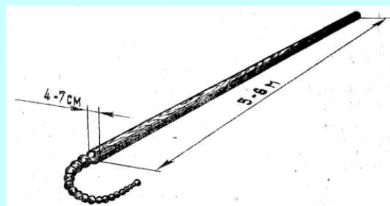
Рис. 10. Спасательный багор
